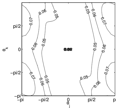
(d) AR = 100, Re = 10000
